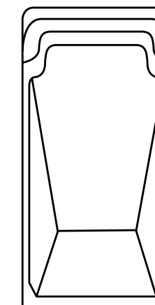
ANAA L 6,50 m x l 3,20 m Prof. 1,40 m Fond plat
